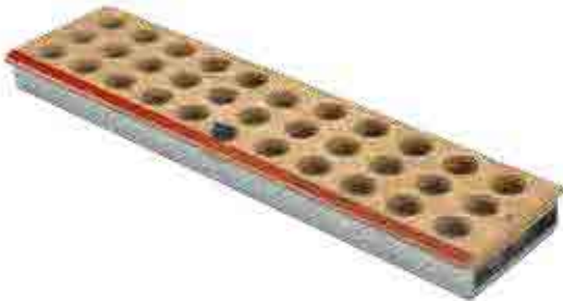
Držák kleštiny ER 32 kompletní
