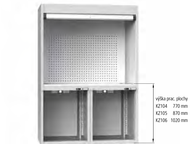
Korpus kontr. pracoviště šířka 1462 mm 36 x 36D
